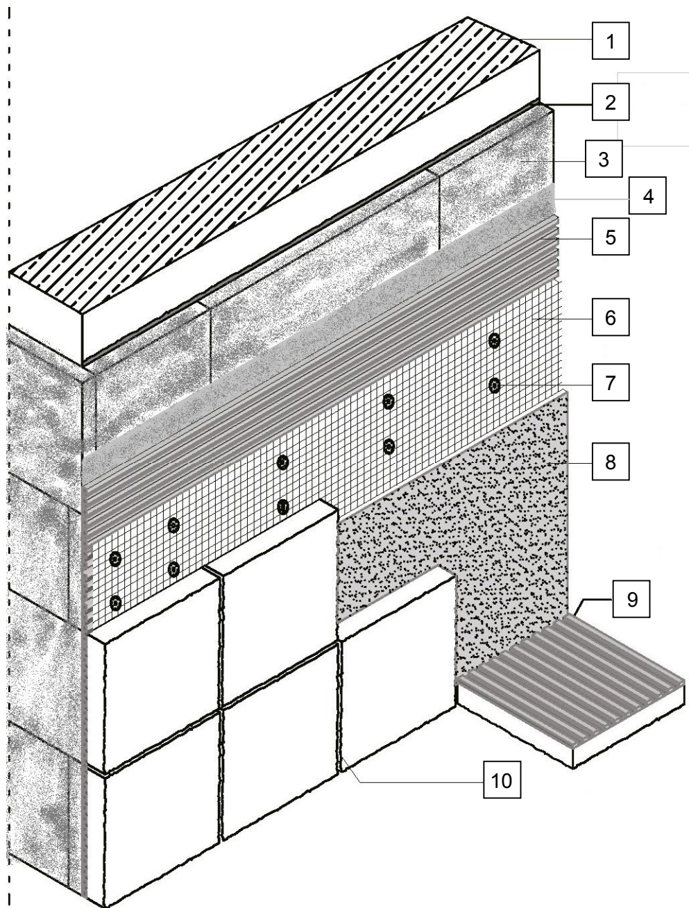
Зображення 1. Пошаровий склад облицьованої теплоізоляційної системи Baunit Star
